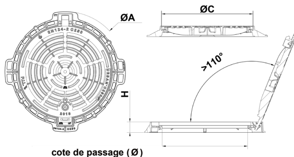
cote de passage (Ø)
